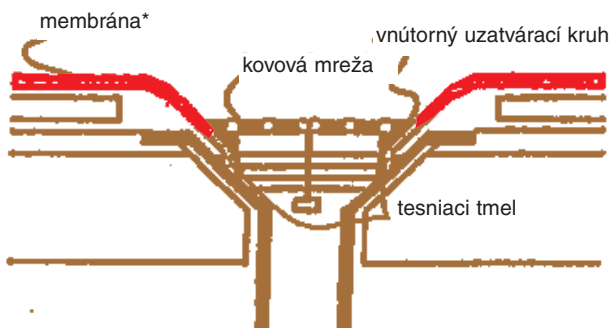
3. Detail strešného odtoku (uzatvorenie kužeľového typu)
