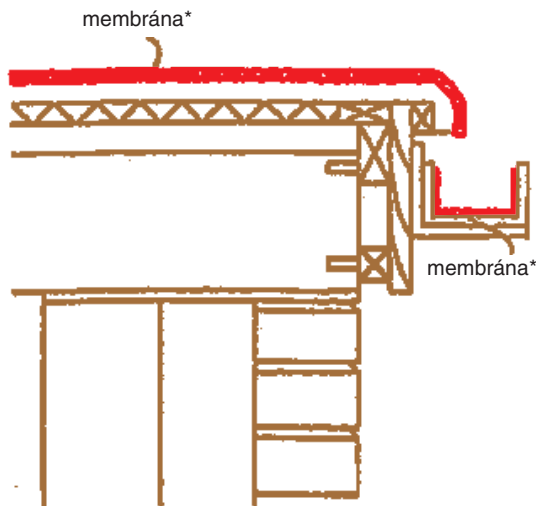
4. Detail okraja k externému odkvapovému žlabu
