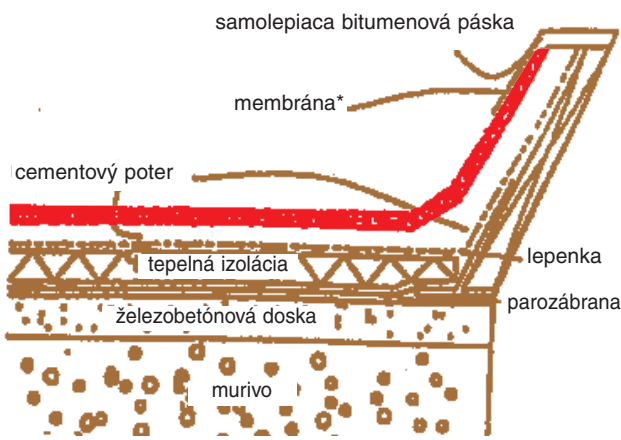
6. Detail lemu vetráka alebo svetlíka
