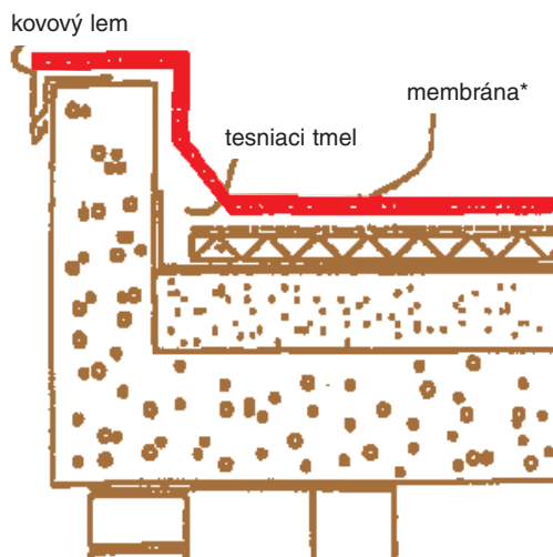
5. Detail obruby s kovovým lemom
