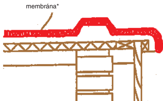
2. Detail okraja s obrubníkom
